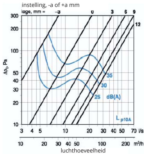
TVR-s/t - 100, 4.5 l/s bij 1 Pa
