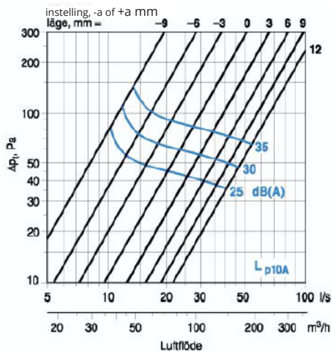
TVR-s/t - 125, 7.0 l/s bij 1 Pa
